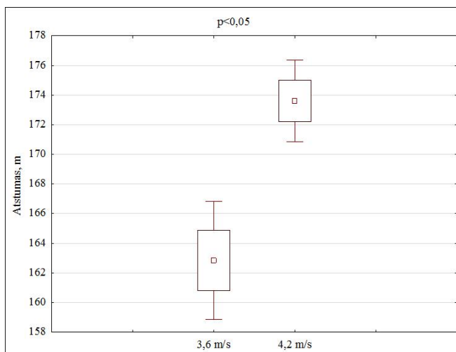
3.3.1 pav. 3,6 m/s ir 4,2 m/s greičio įtaka maršruto efektyviam ilgiui per minutę
